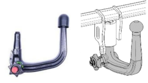
Szerszám nélkül leszerelhető vonóhorog 13 pólusú csatlakozóval
